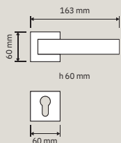
1055 FP Pomolo fisso con placca / Fixed knob on plate
