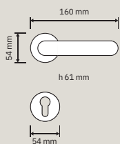
1055 PT 070 Pomolo a tirare / Fixed knob
